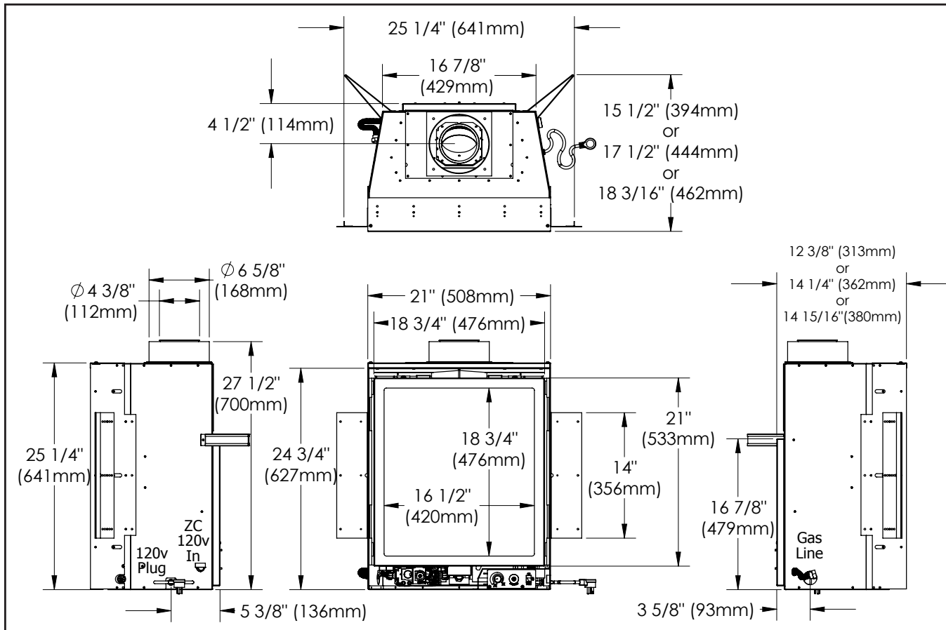
Figure 1. Q1CI Dimensions - Top Vent
