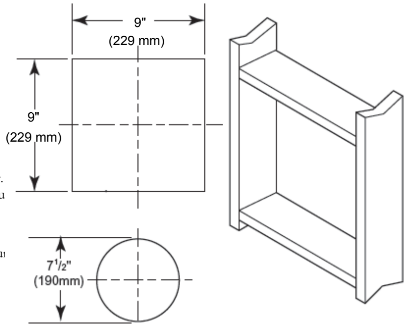
Schéma 12 - Exigences pour l'ouverture du système d'évacuation
