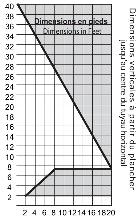
Schéma 10 – Graphique du Mur Arrière du Système d'Évacuation
