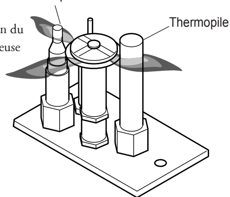
Schéma 52 - La flamme de la veilleuse
