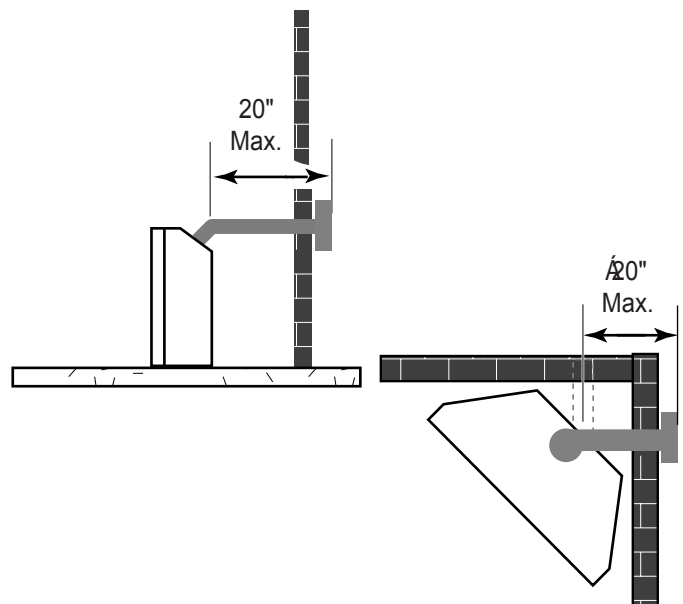
Schéma 19 – Conduit horizontal maximum sans élévation
