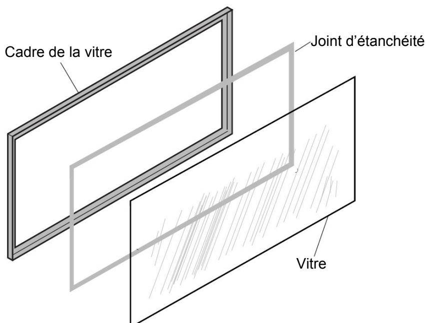
Figure 38 – Remplacement de la vitre (vue de l'intérieur du cadre)
