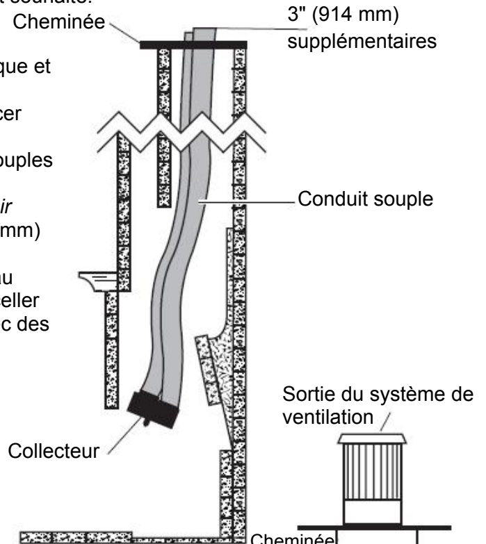
Figure 9 – Fixer le conduit souple au collecteur
