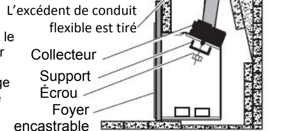
Figure 11 – Glisser le foyer en place.
