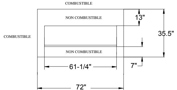
INSTALLATION ENCASTRÉE
