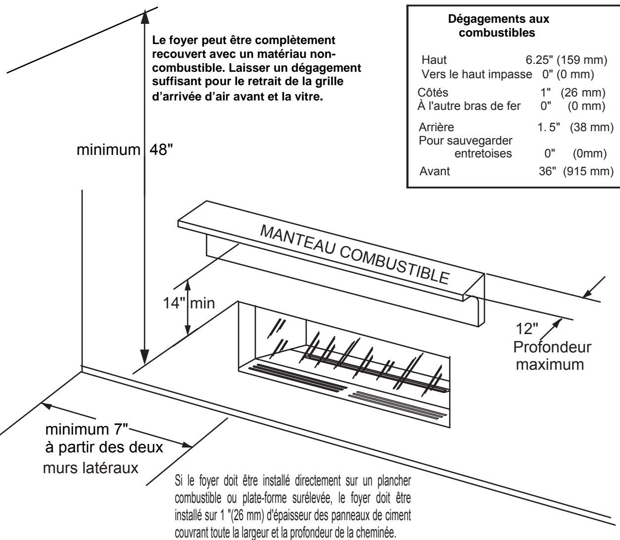
Schéma 6 - Dégaquements
