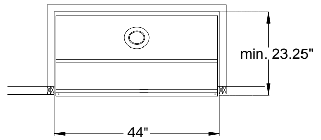
Schéma 2 – Dimensions d'encadrement
