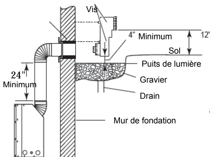
Schéma 23 – Installation sous le niveau du sol
