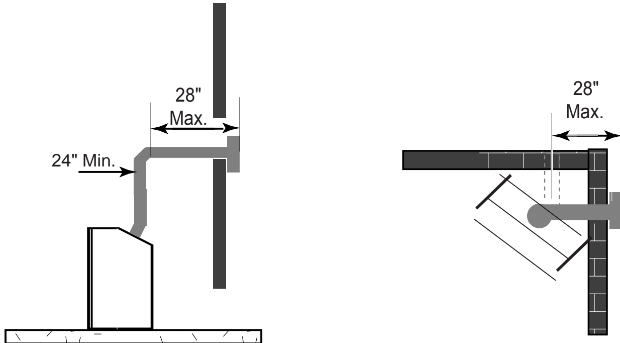
Schéma 19 – Parcours maximum horizontal sans élévation
