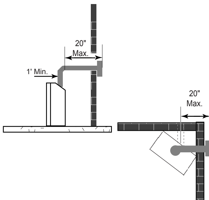
Schéma 19 – Parcours maximum horizontal 3' élévation
