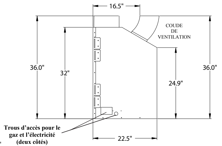
VUE DU CÔTÉ DROIT avec coude de 30 degrés
