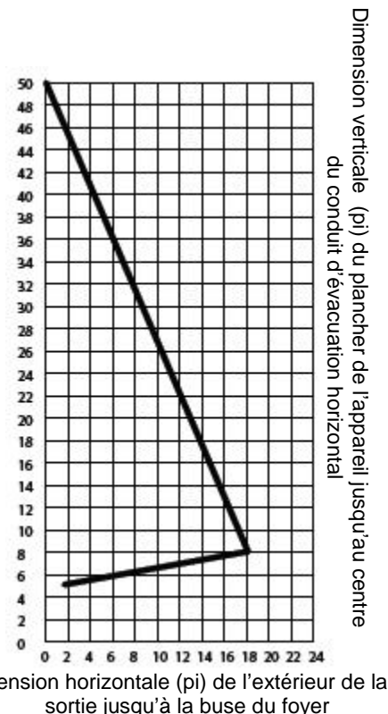
Schéma 10 – Graphe de configurations de ventilation autorisées
