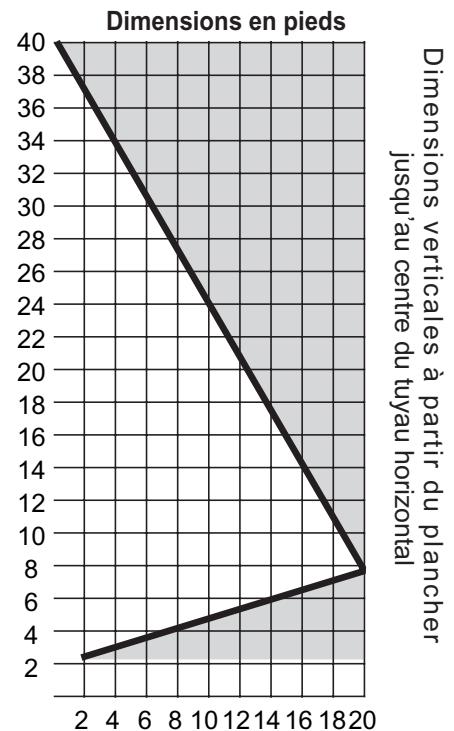
Schéma 9 - Tableau des distances permises pour l'évacuation
