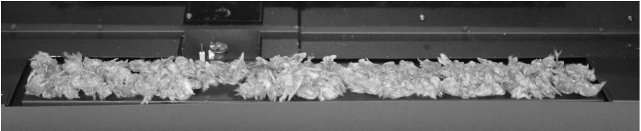
Figure 37 - Placement de la laine de roche sur Burner
