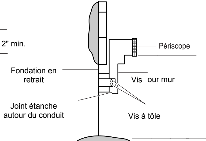
Schéma 24 – Installation du périscope, fondation en retrait
