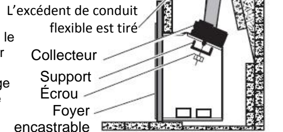
Figure 10 – Glisser le foyer en place.
