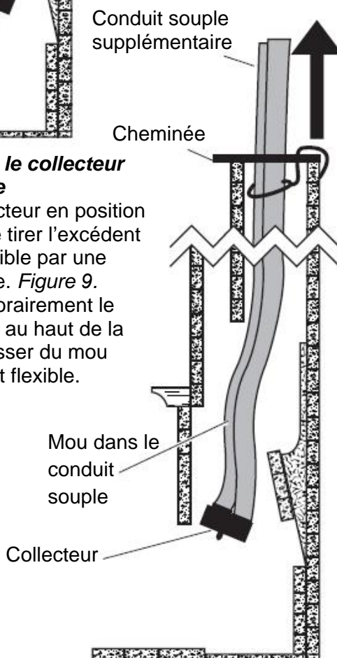
Figure 9 – Tirer l'excédent de conduit
