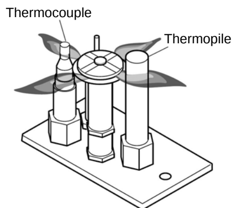
Figure 34 – Apparence normale de la flamme de la veilleuse
