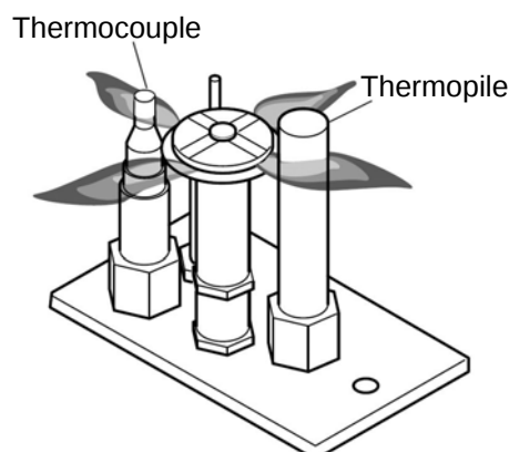
Figure 35 – Avant de démonter l'appareil, vérifier la flamme de la veilleuse. La flamme doit toucher le thermocouple et la thermopile.
