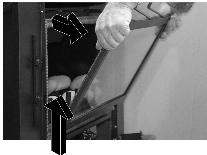
Figure 24 - Retrait de la porte en verre
