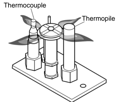
Figure 35 – Avant de démonter l'appareil, vérifier la flamme de la veilleuse. La flamme doit toucher le thermocouple et la thermopile.
