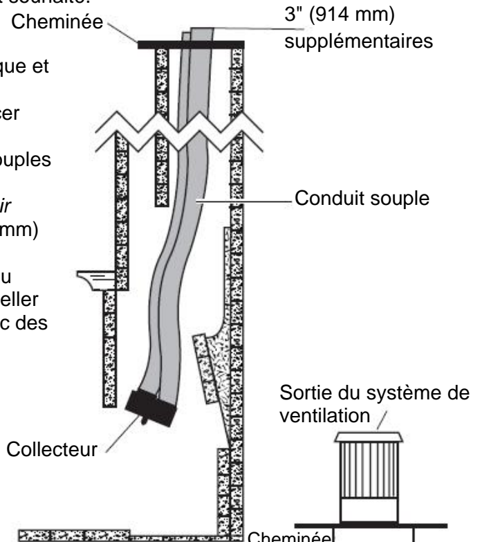
Figure 8 – Fixer le conduit souple au collecteur
