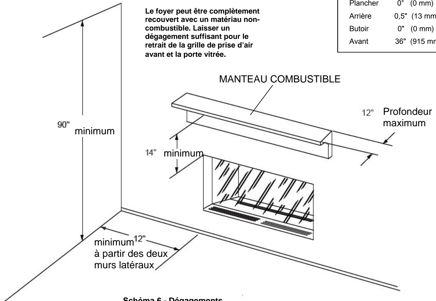
Schéma 6 - Dégagements
