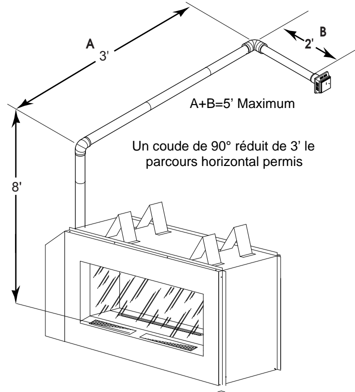
Schéma 20 – Réduction de parcours horizontal
