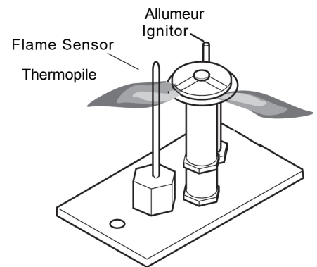
Schema 45 - L'appareil Flamme
