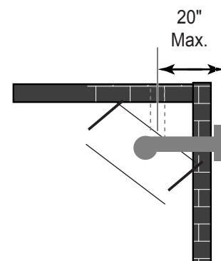
Schéma 19 – Parcours maximum horizontal 3' élévation
