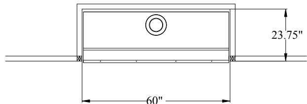
Schéma 2 – Dimensions d'encadrement
