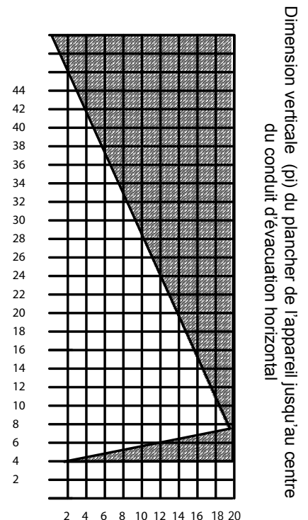
Dimension horizontale (pi) de l'extérieur de la sortie jusqu'à l'arrière du foyer
